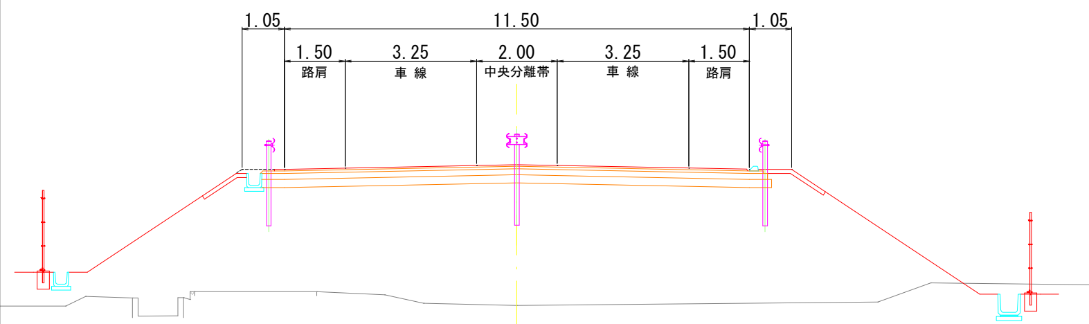
○断面図 土工部 (一般道側ランプ) 単位：m
