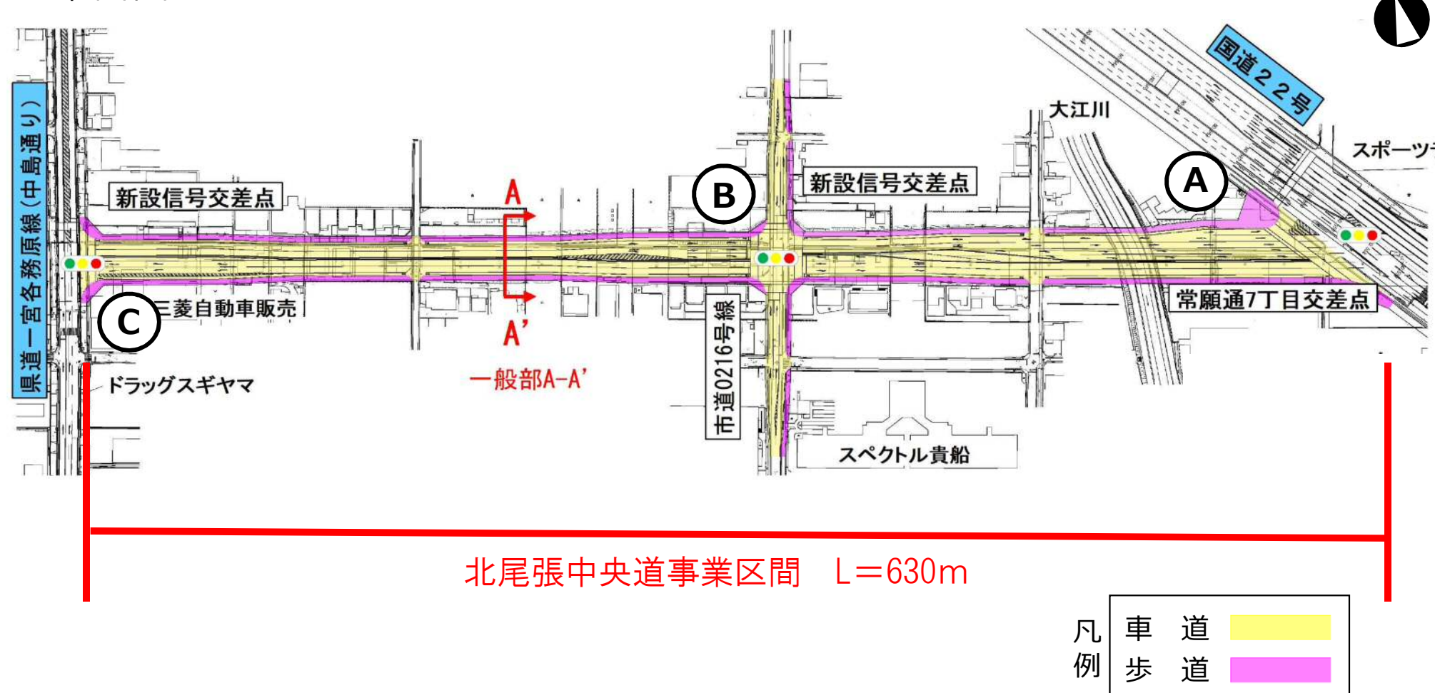
○平面図
